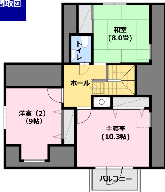
2F間取図
